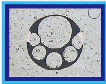
共押出マルチルーメンチューブ (非対称)
