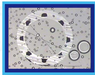
OD 0.3mm 静脈用PU チューブ (造影剤入)
